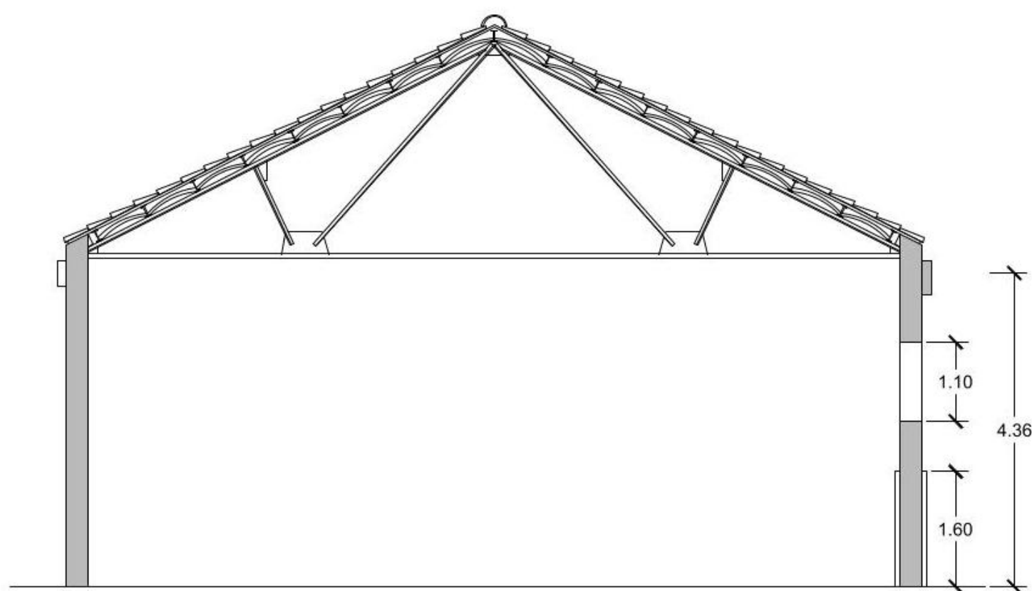
Secció 1
