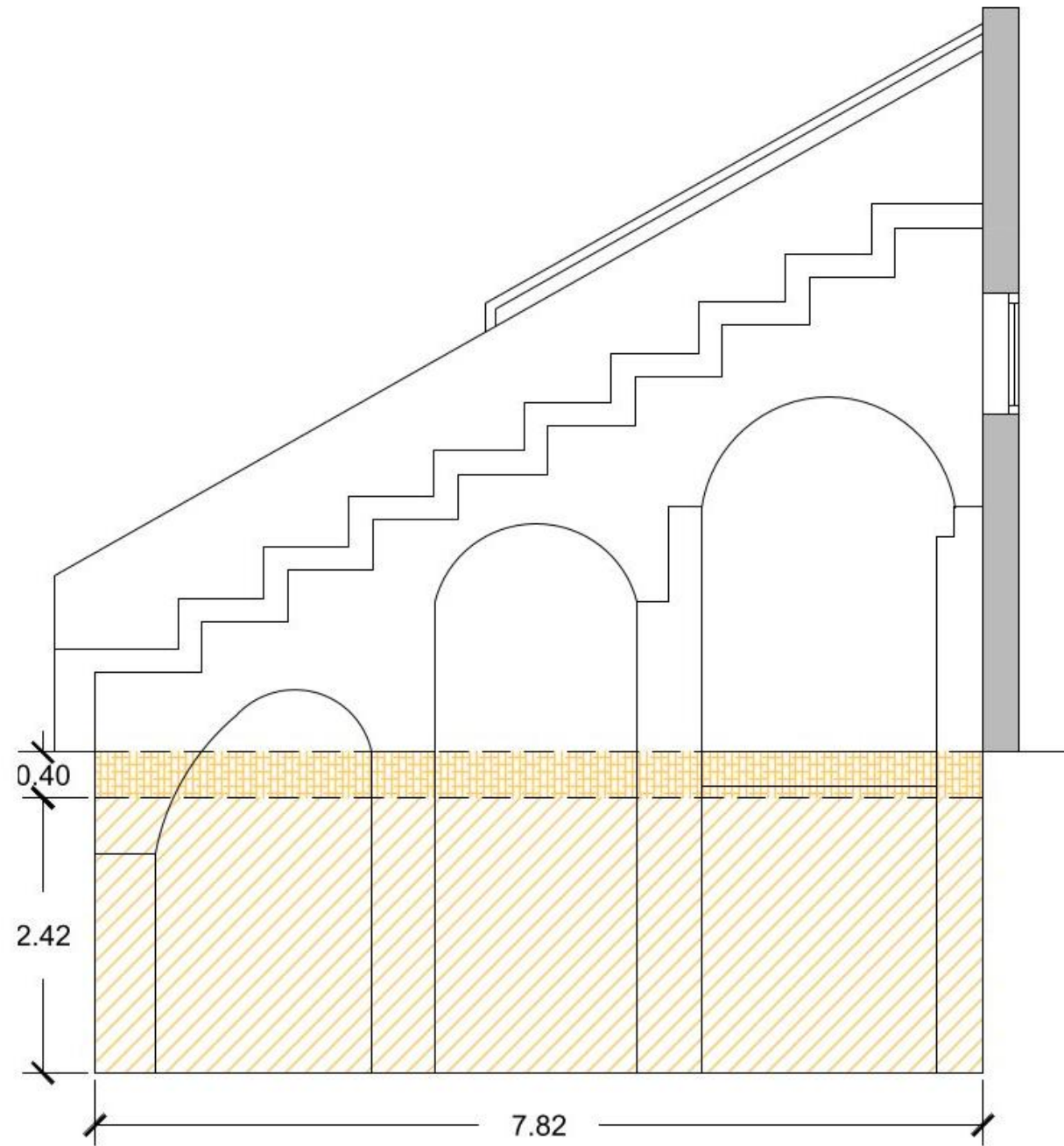
Secció 2
