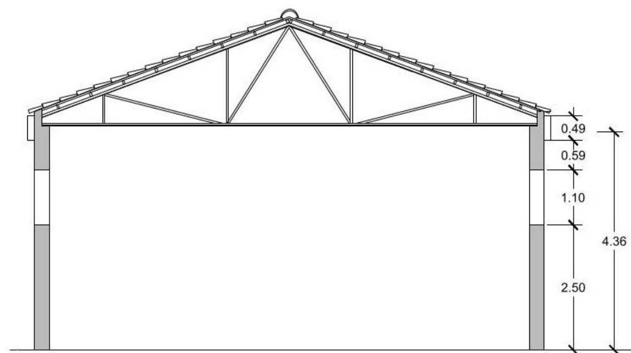
Secció 2
