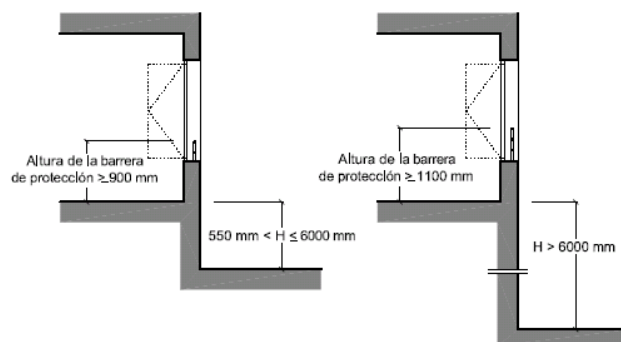
Figura 3.1. Barreras de protección de ventanas
