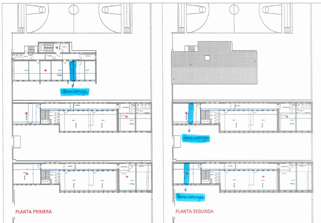
Plano de ubicación de las 3 pruebas de carga realizadas en los dintinto forjados de los edificios
