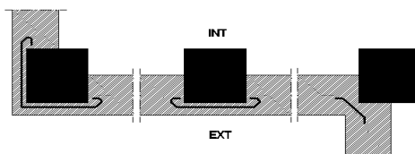
Figura 2.9 Ejemplo de encuentro de la fachada con los pilares
