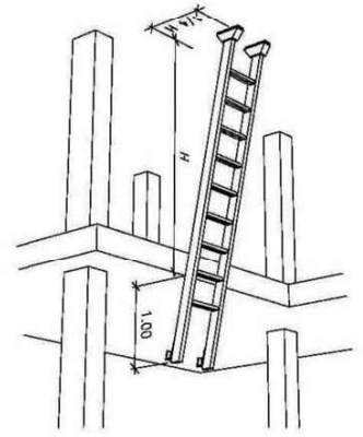
POSICIÓN CORRECTA DE ESCALERAS DE MANO
