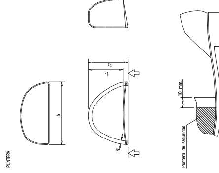
PROTECCIONES INDIVIDUALES (BOTAS DE SEGURIDAD - REFUERZOS - )
