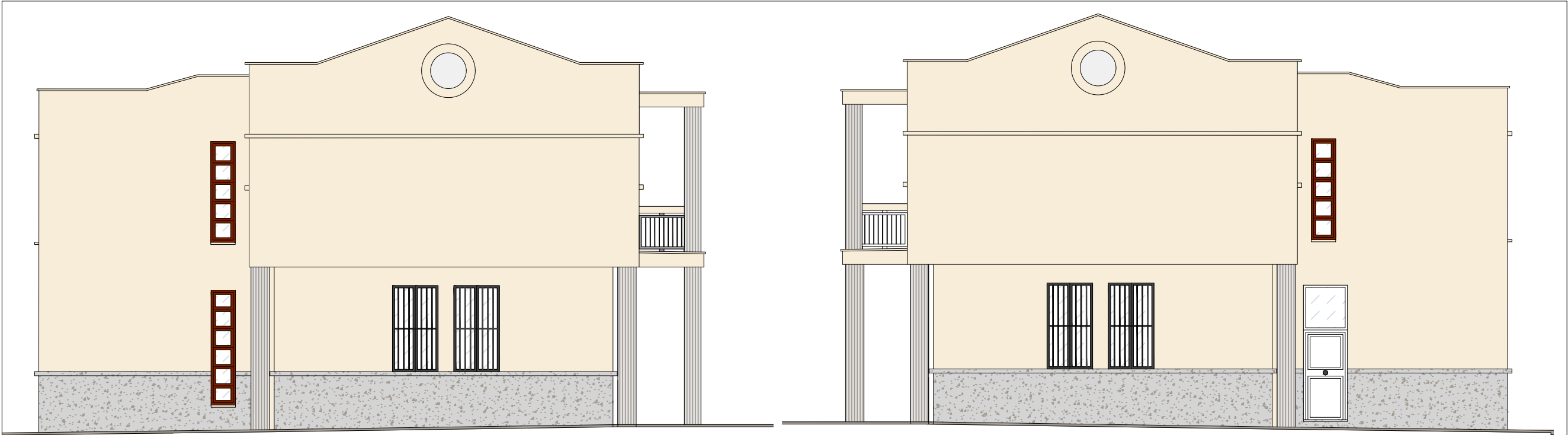
FAÇANA NORD-EST
