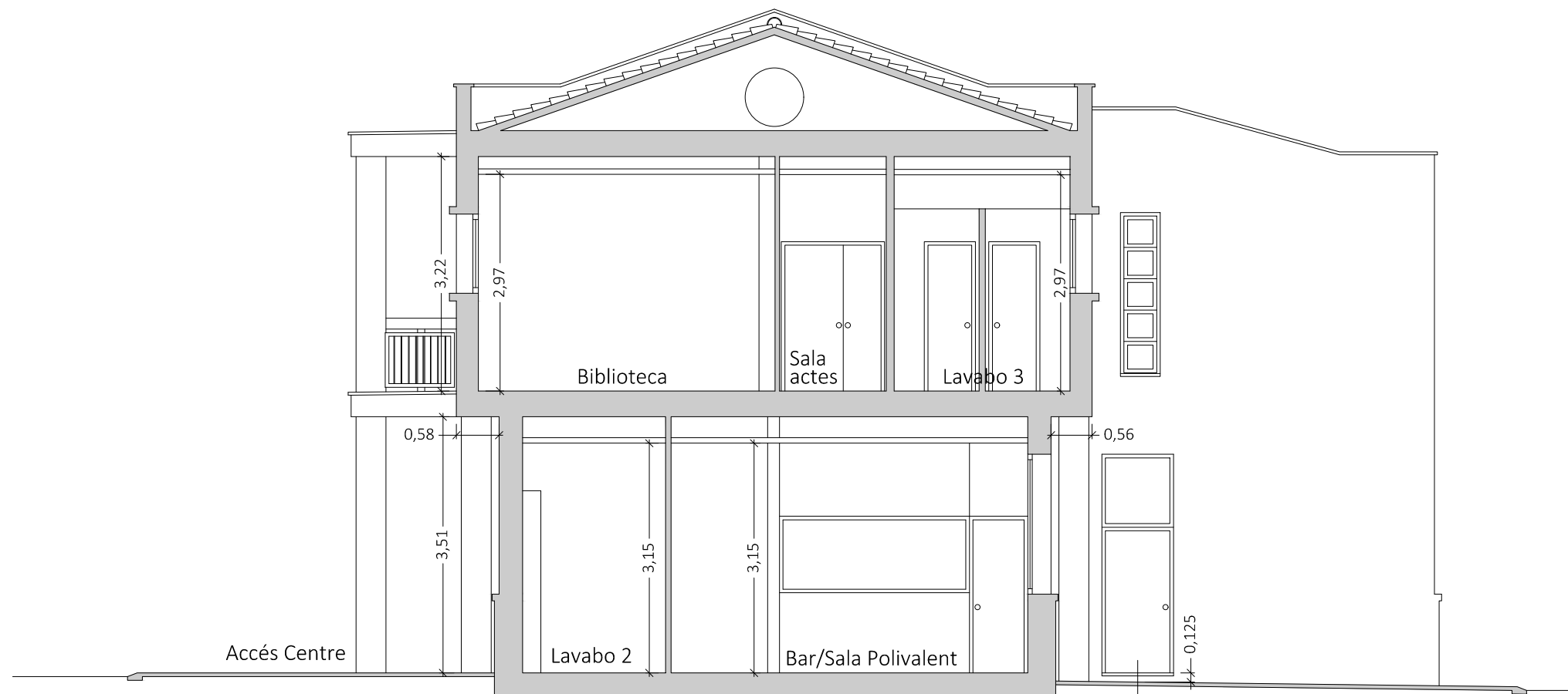
SECCIÓ B-B'
