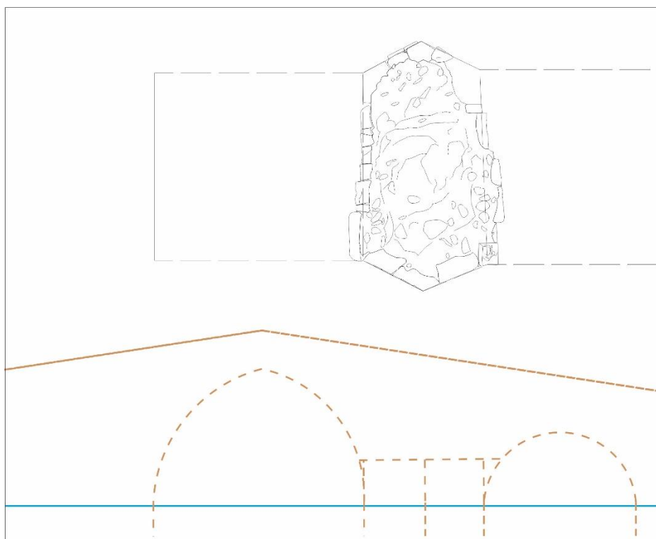
Planta de l'estrep del pont i proposta de restitució del funcionament amb la línia del nivell del riu.
