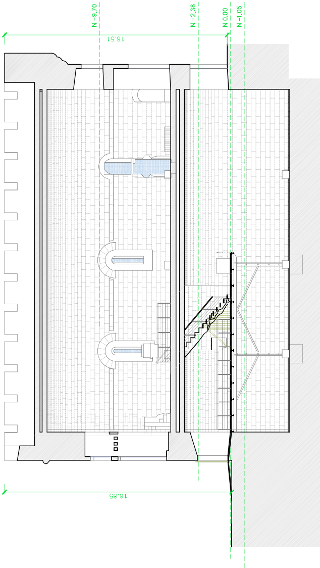
SECCIÓ A-A
