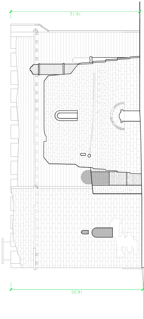
FAÇANA OEST
