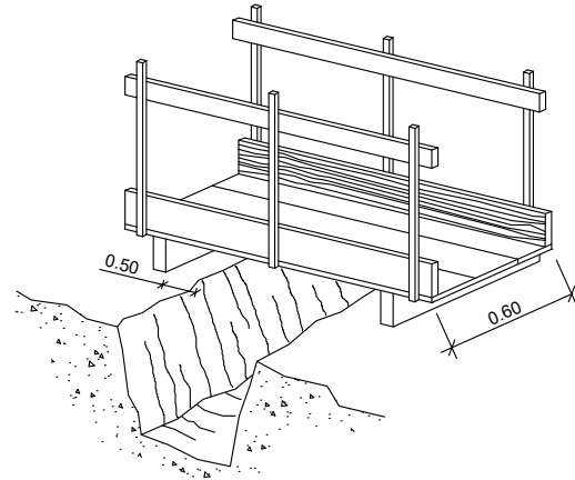
DETALL DE PASSARELLA VIANANT
