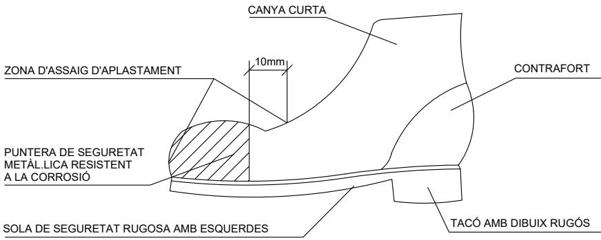
BOTA DE SEGURETAT CLASSE III
