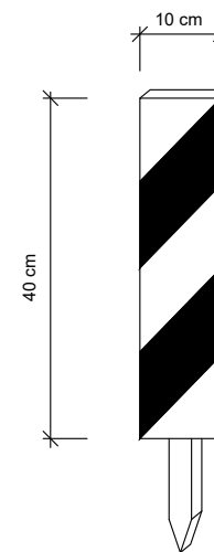
PIQUETA 10x10x40
