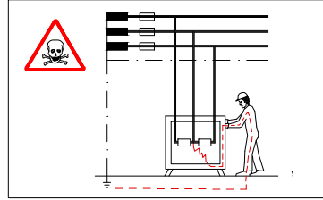
DEFECTES D'A LLAMENT EN MÀQUINES SENSE PROTECCIÓ.
