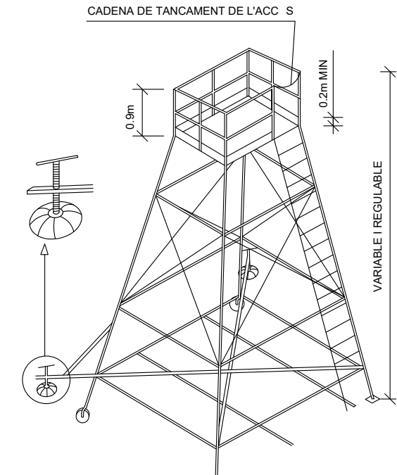
TORRETA
