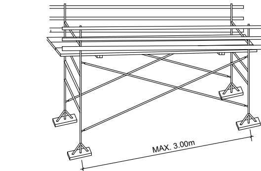
PLATAFORMES DE TREBALL METÀL·LIQUES
