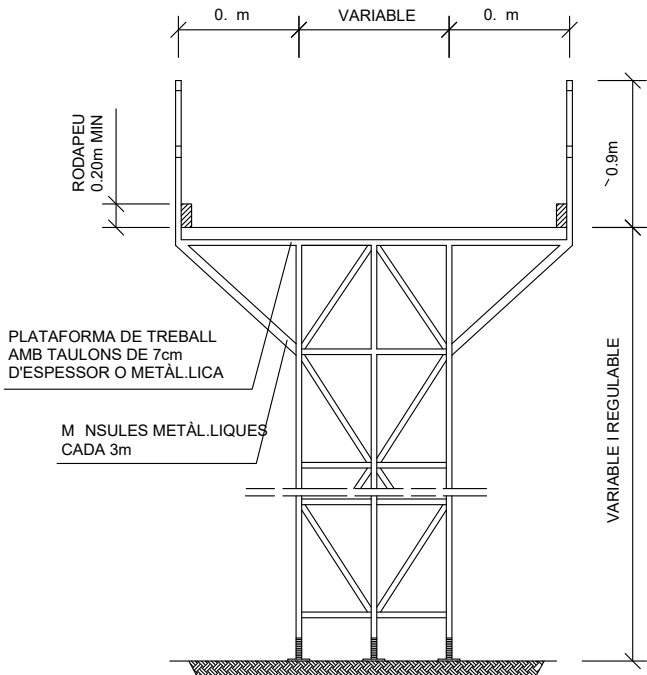
BASTIDA METÀL·LICA
