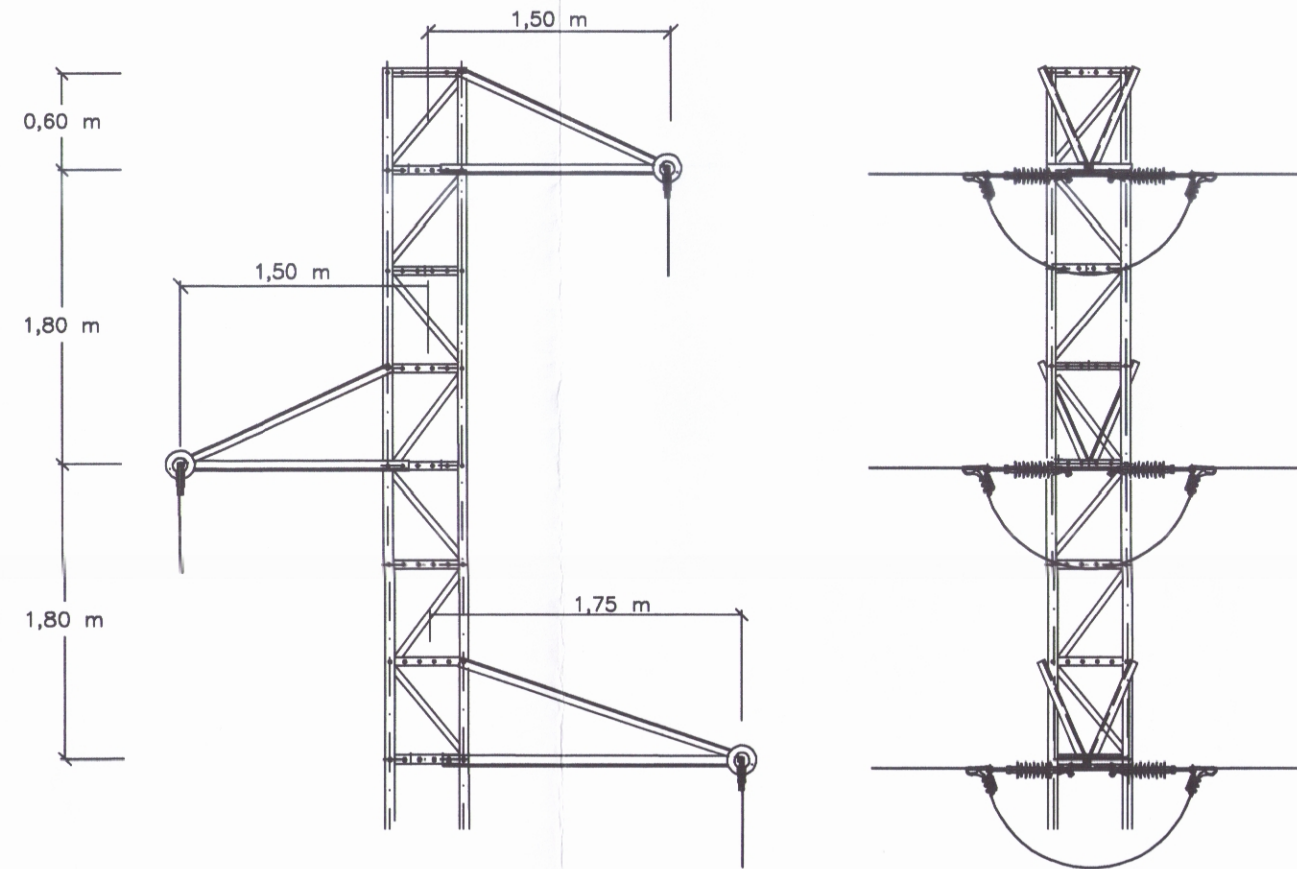
ARMAT Montseny L Amarre (detall armat dels suports N° 2 i 3)
