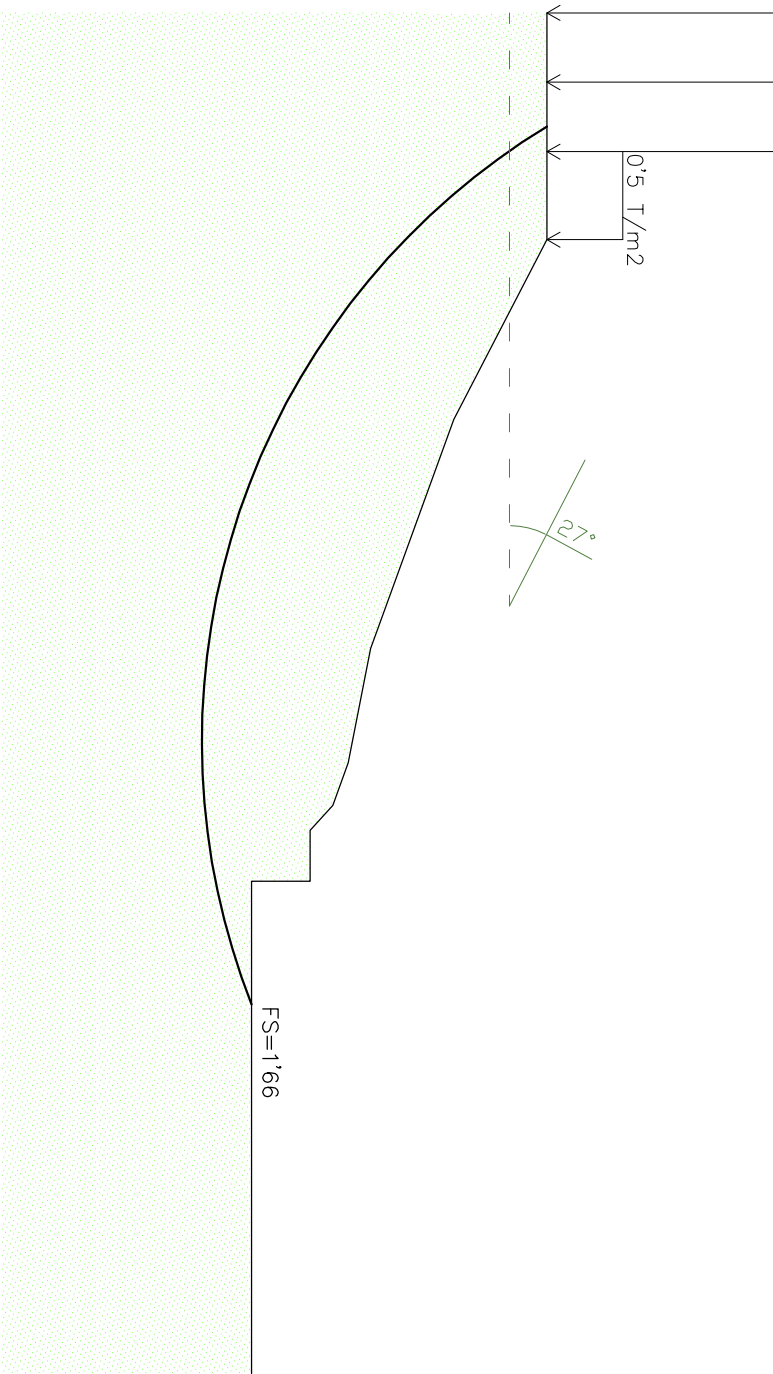
Secció S23
