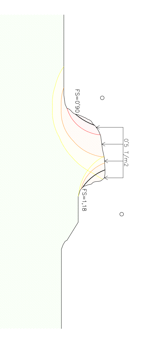
Secciò S30
