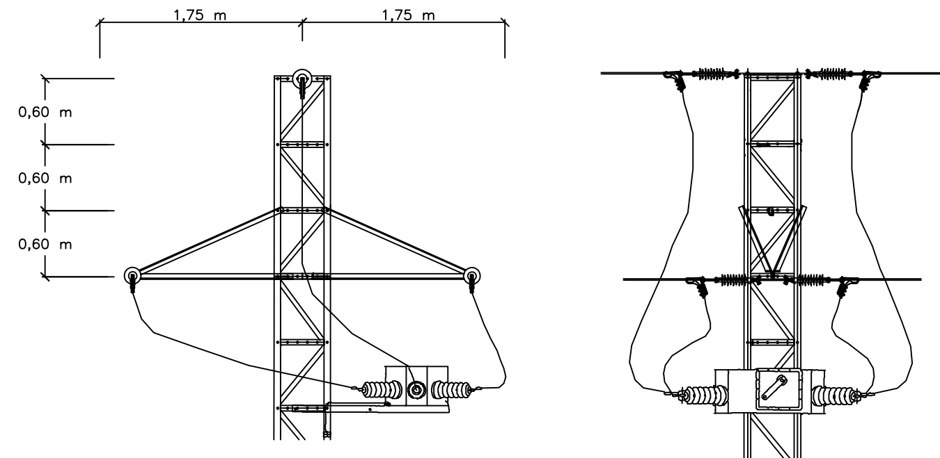
ARMAT TRIANGLE AMARRE (TR2 Pos 3) + SECCIONAMENT III SF6 (detall armat del suport N° 1)
