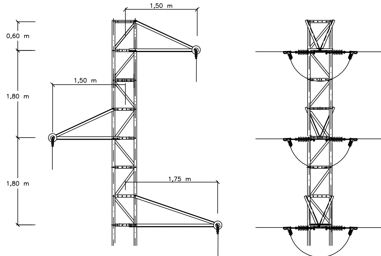
ARMAT Montseny L Amarre (detall armat dels suports N° 2, 3, 4, 5 i 6)
