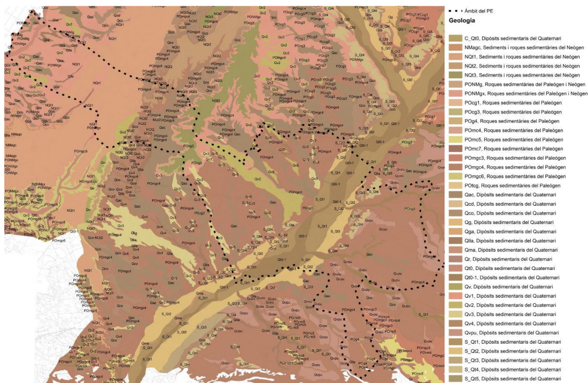
Figura 3. Geologia de l'àmbit d'estudi i entorns
