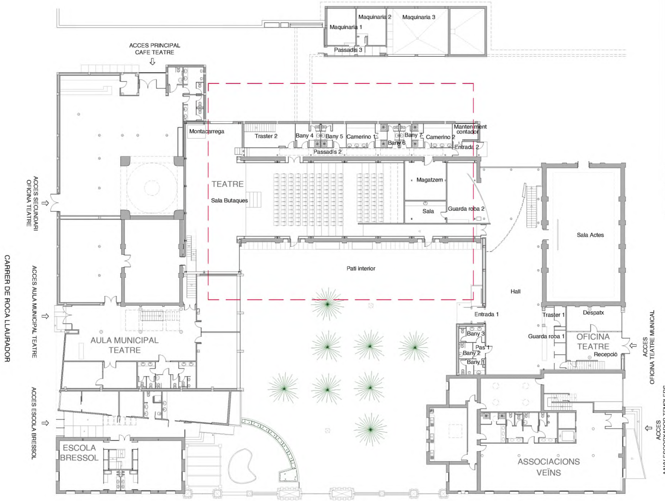
Planta baixa
