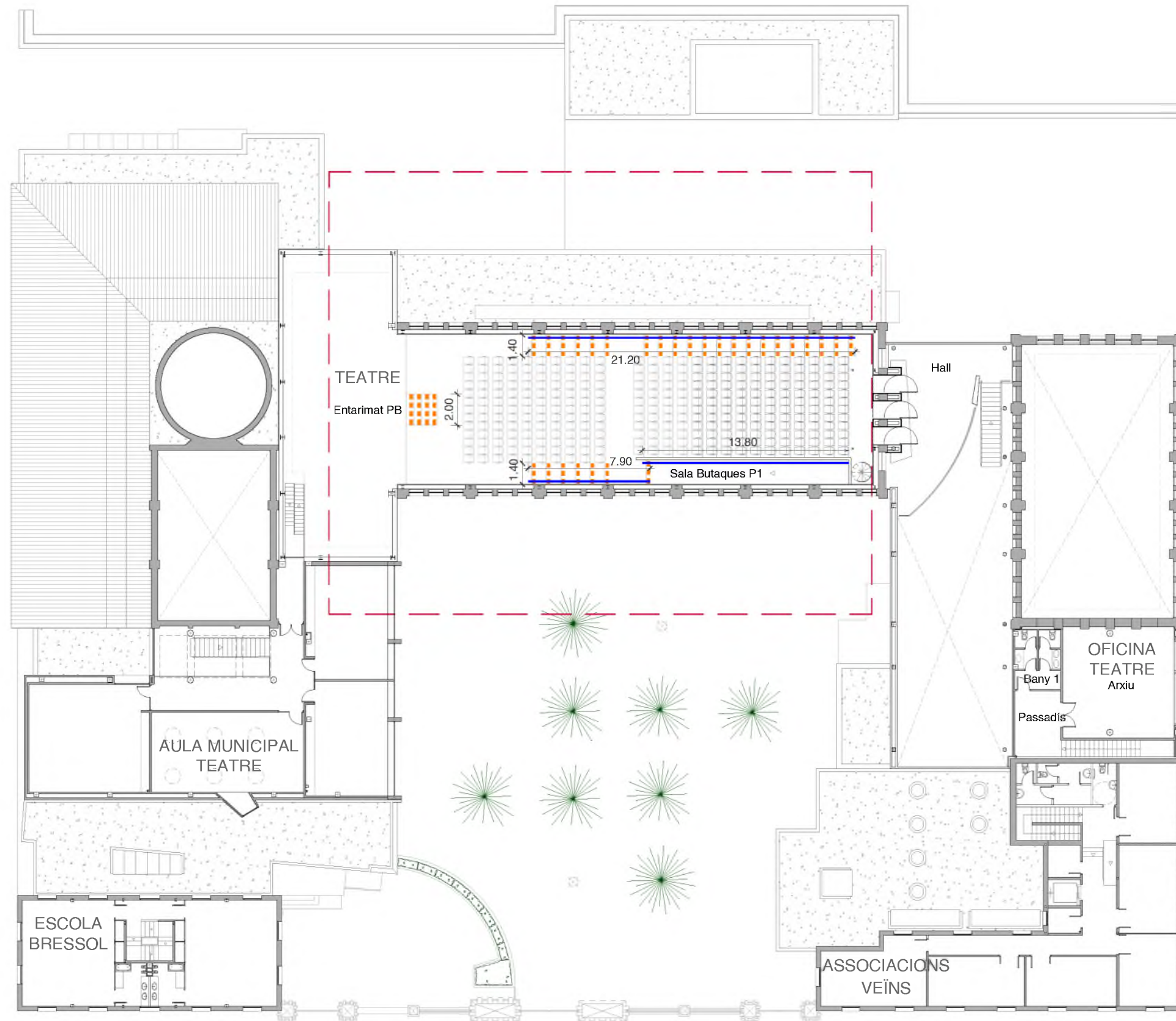
Planta primera
