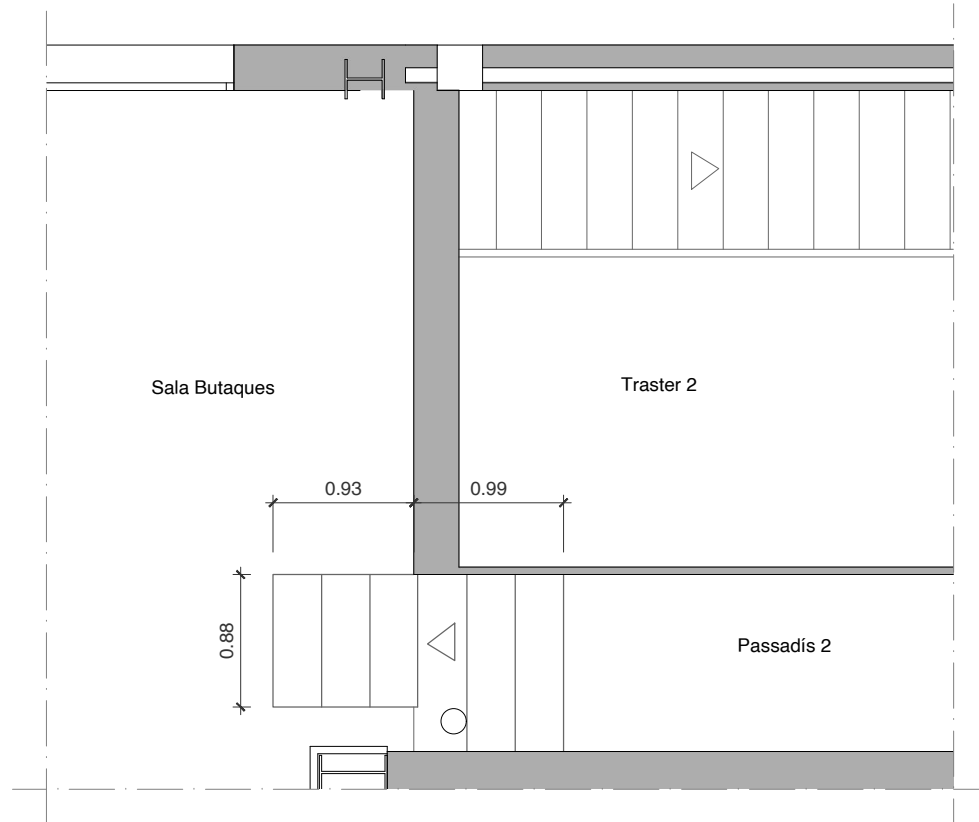
Planta
