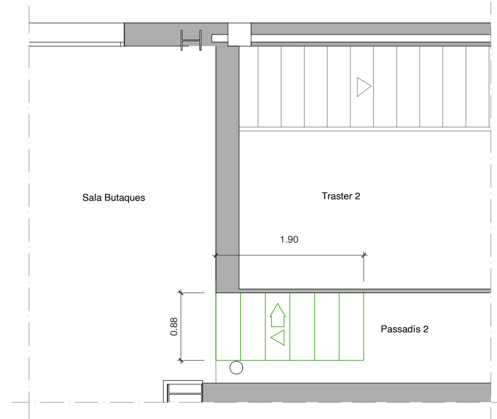
Planta
