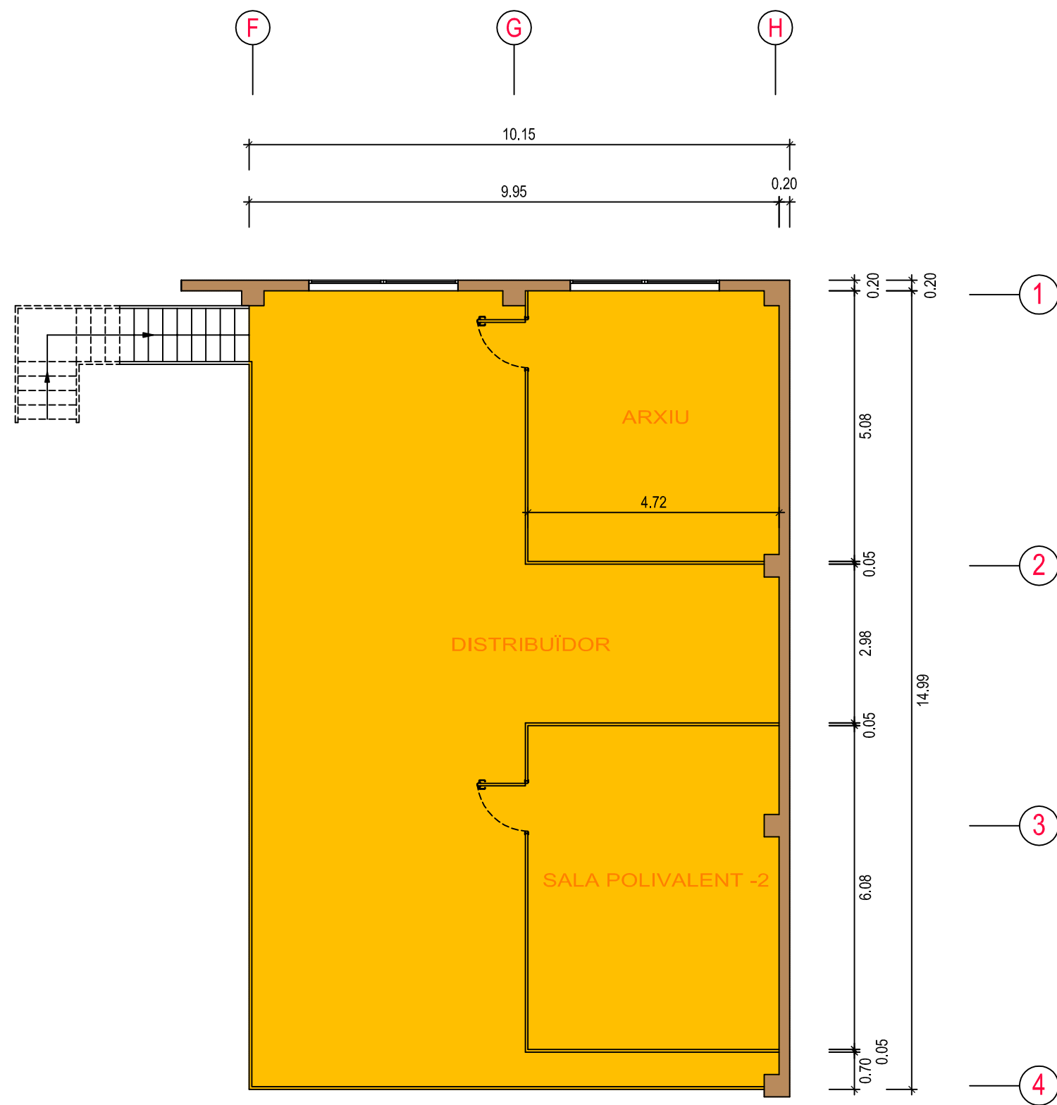
PLANTA GENERAL DISTRIBUCIÓ I COTES. PLANTA ATELL E.- 1/100
