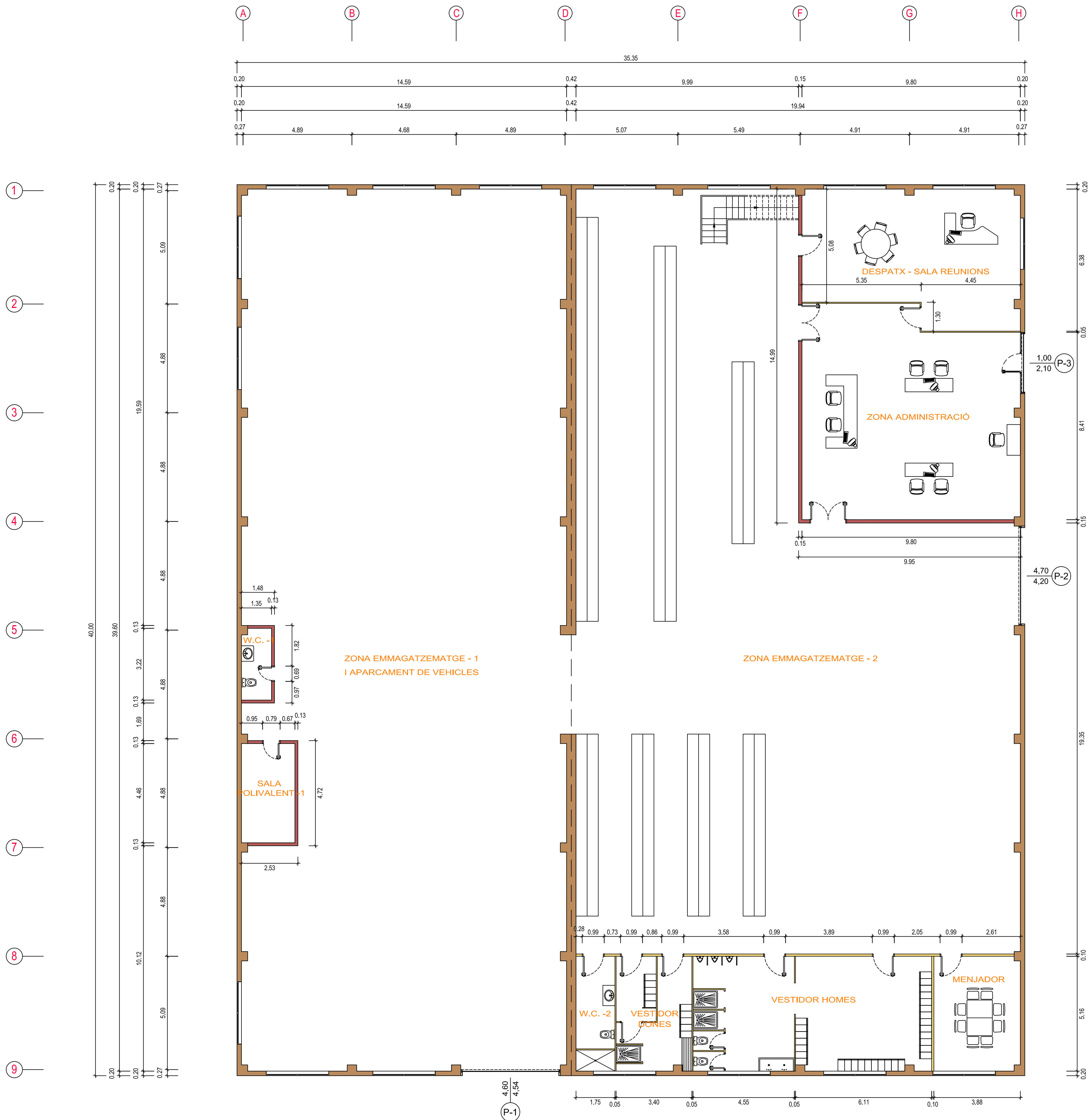
PLANTA GENERAL DISTRIBUCIÓ I COTES E.- 1/100
