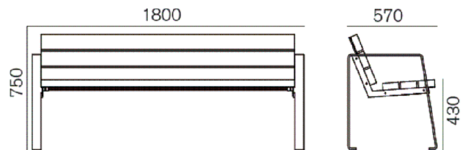
Banco modelo Equus Technical Wood o similar de 1800 mm de longitud
