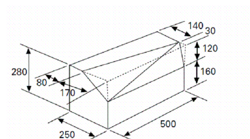
DETALLE BORDILLO TRANSICIÓN GUAL PEATONES Y VEHICULOS
