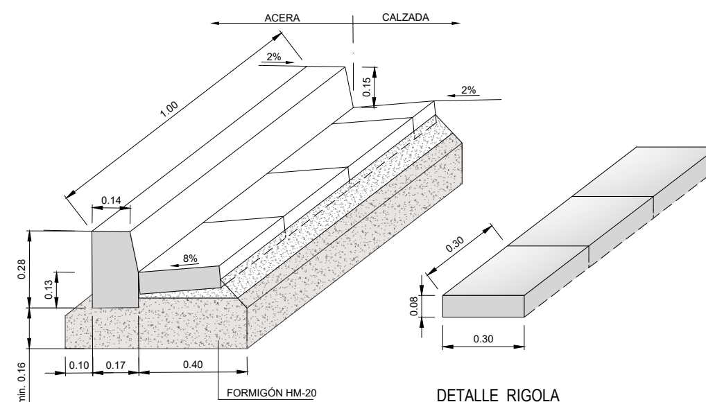
DETALLE BORDILLO TIPO C3 CON RIGOLA
