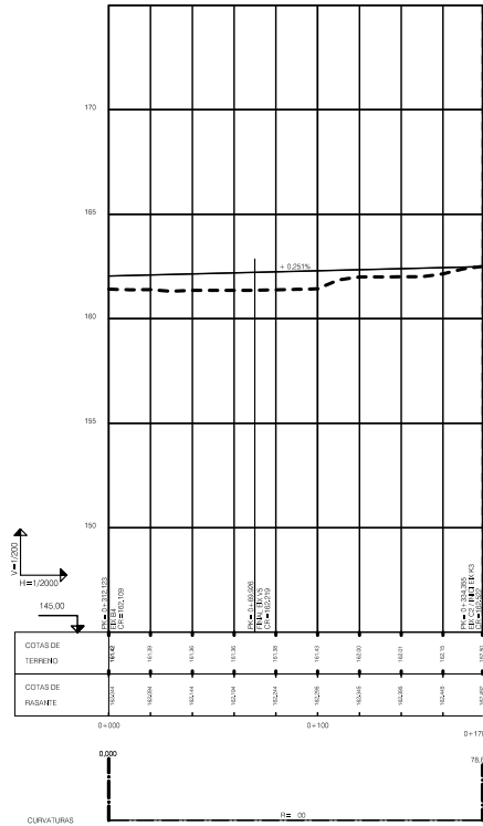
PERFIL LONGITUDINAL EIX K2
