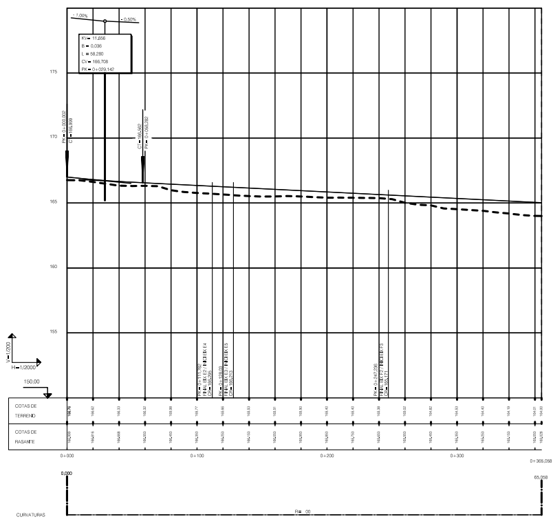
PERFIL LONGITUDINAL E1 E1: 1000 E2: 1000 E3: 1000
