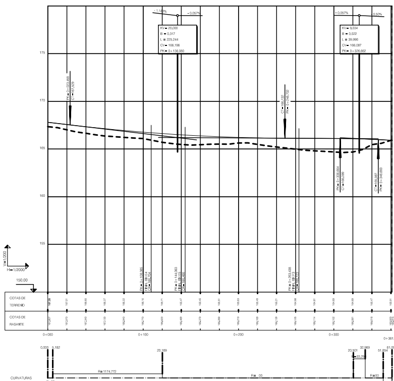
PERFIL LONGITUDINAL E3 E1: 1000 E2: 1000 E3: 1000
