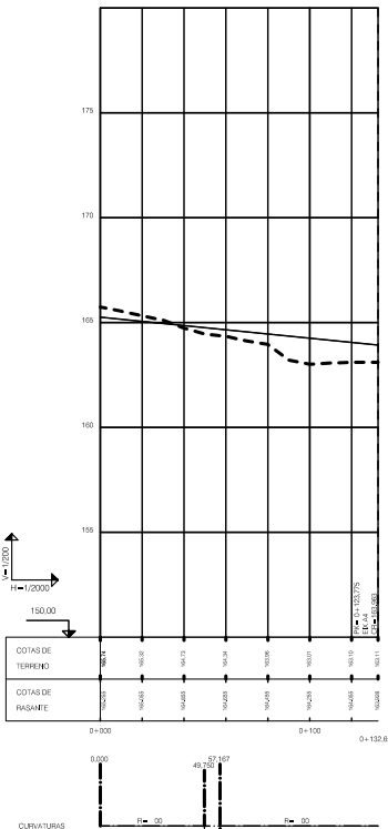
PERFIL LONGITUDINAL EIX P7
