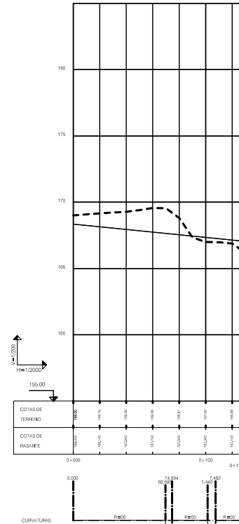
PERFIL LONGITUDINAL EIX P5
