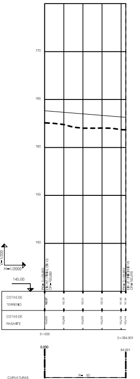
PERFIL LONGITUDINAL EIX V4
