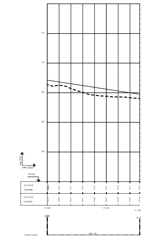
PERFIL LONGITUDINAL E10 E1: 1000 E2: 1000 E3: 1000
