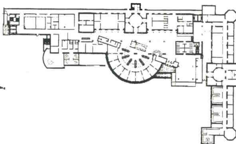
Planta Baixa. Hospital - CAP.
