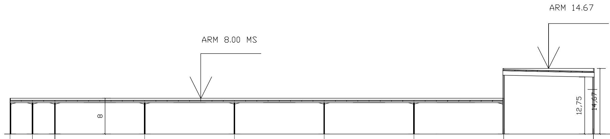
SECCIÓN B-B
