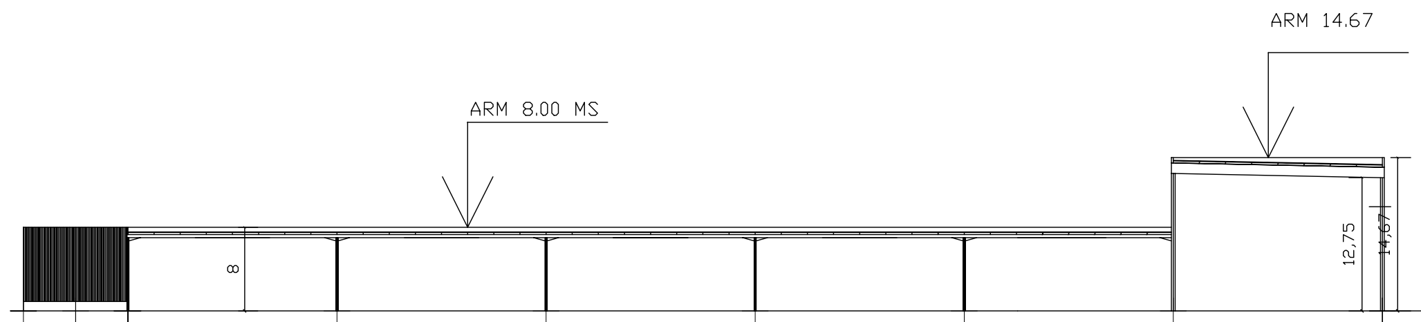
SECCIÓN A-A
