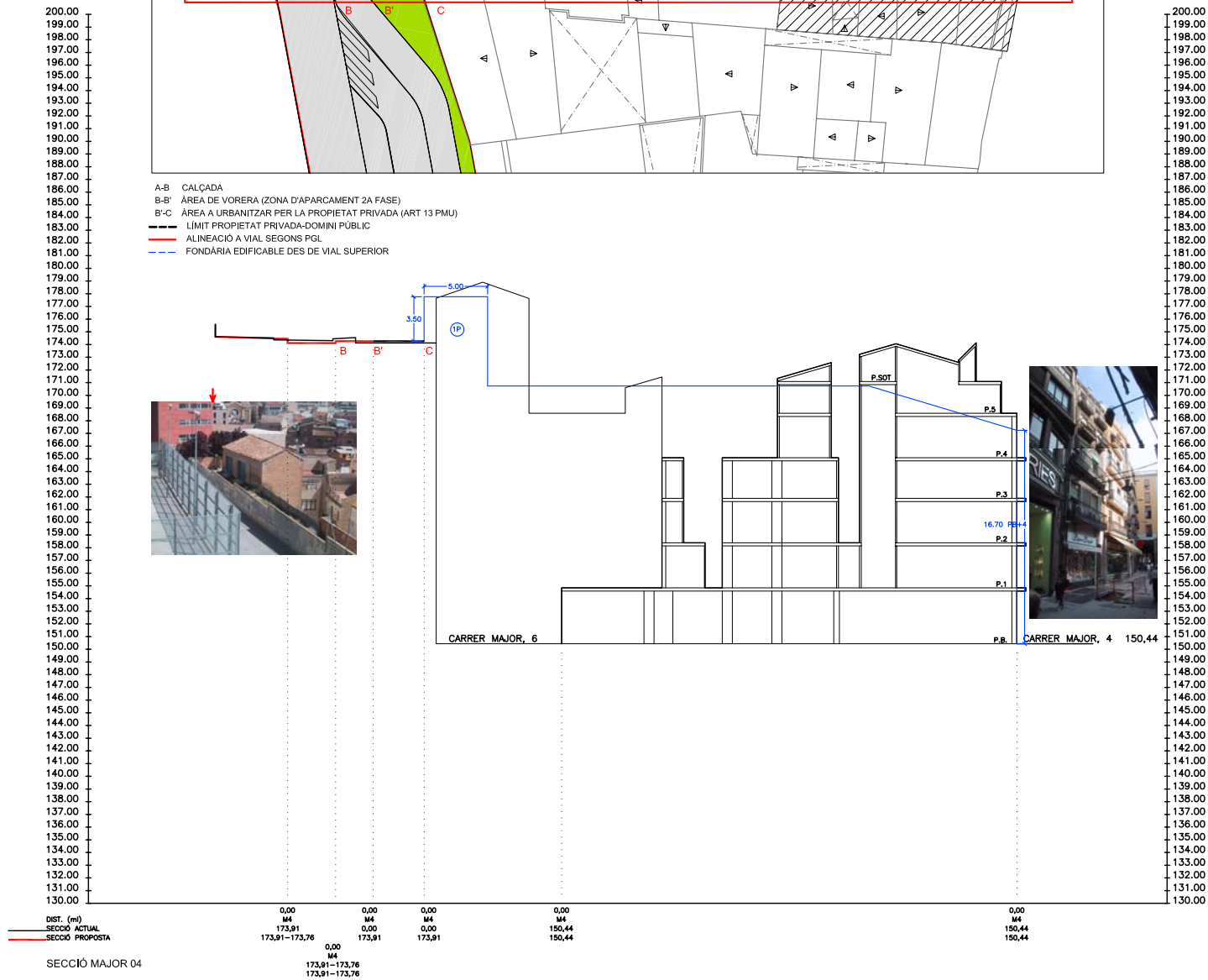
SECCIÓ MAJOR 04
