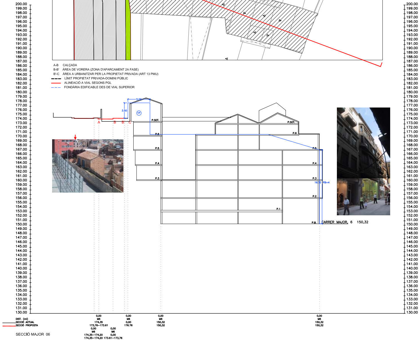
SECCIÓ MAJOR 06
