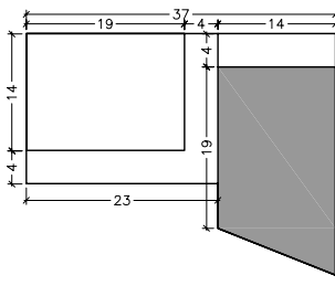
PLANTA NIVELL 183.90
