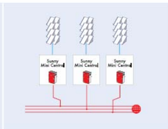
Ejemplo de cableado del Sunny Mini Central (conexión a red trifásica)
