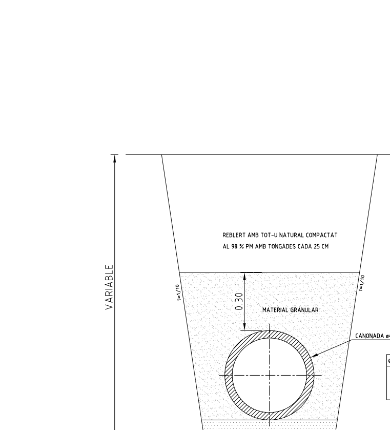
RASA TIPUS e 1/20
