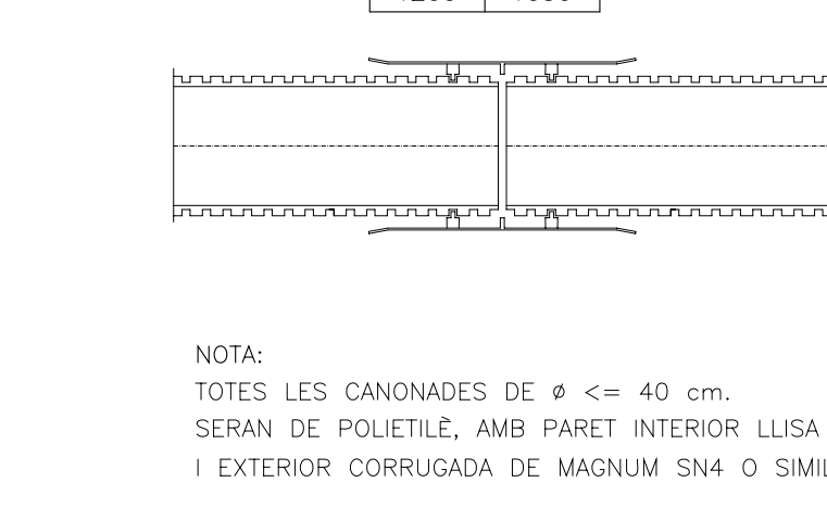
CANONADA DE POLIETILE SN4 AMB JUNTA H/H
