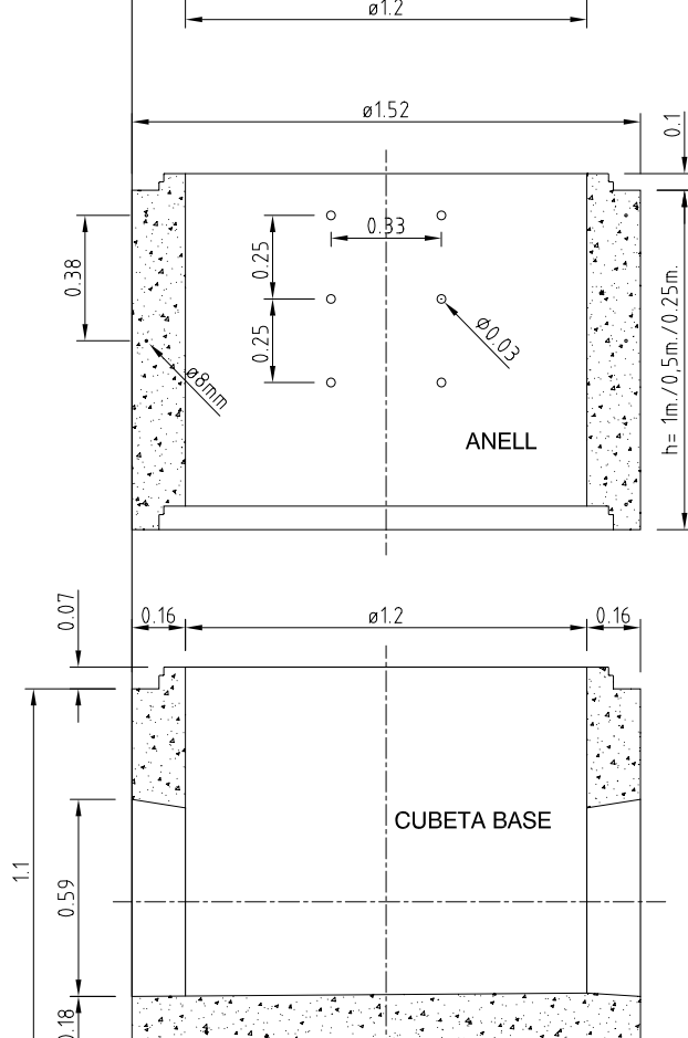
POU DE REGISTRE e 1/25
