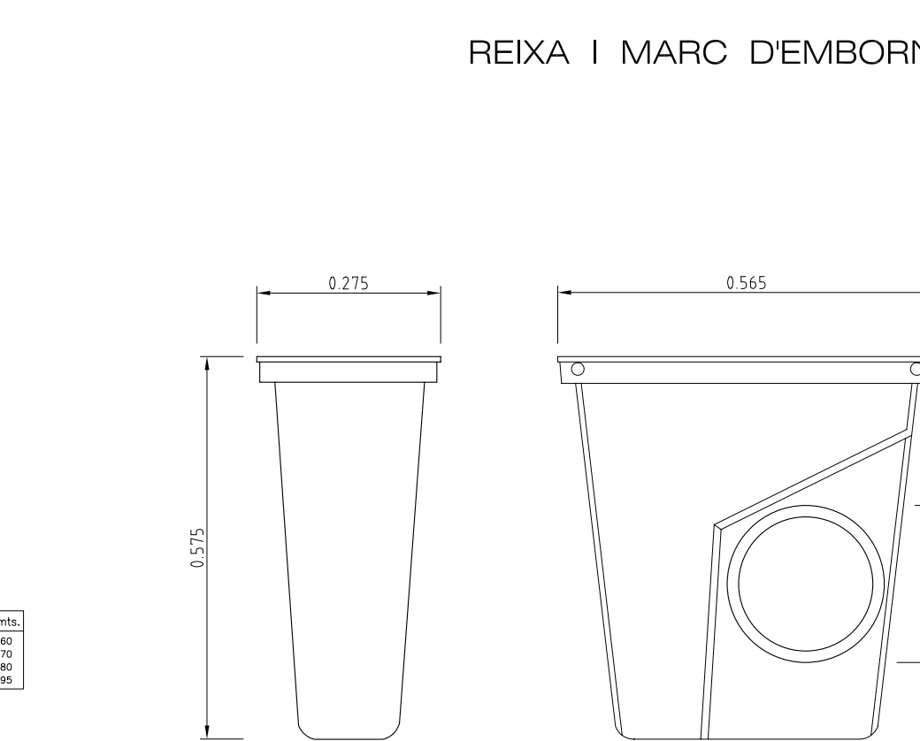
EMBORNAL TIPUS DELTA SF570 e 1/10
